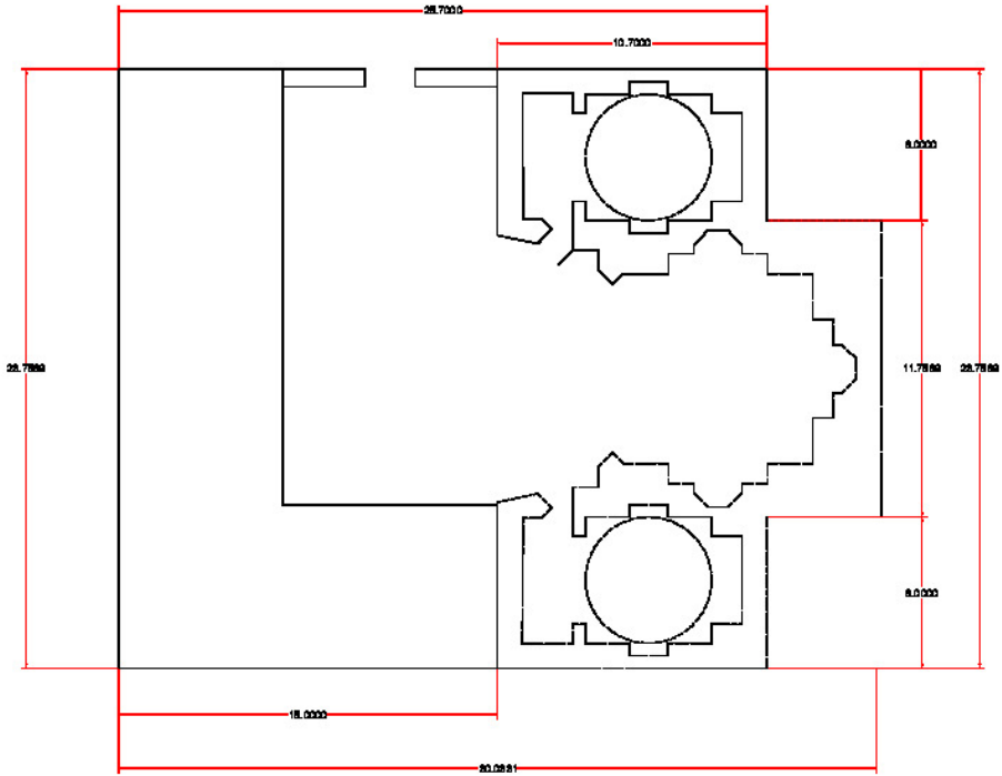
پلان ۲: نقشه احتمالی بنای ساخته شده دوره تیموری خانقاه جلال الدین بایزید پورانی (ایوان اصلی و دو اتاق مجاور)
